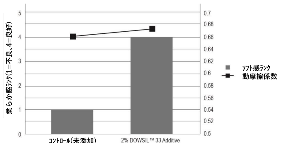
図 1: プラスチック用 2 液型ウレタンコーティングへの DOWSIL™ 33 Additive 添加によるソフト感付与効果と動摩擦係数の評価結果。ソフト感ランク(1~4): 1=不良 ~ 4=良好。動的摩擦係数の値は DOWSIL™ 33 Additive を配合しても低下しないことを示しています。
