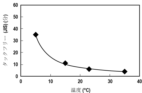
図 1: 表面硬化性
