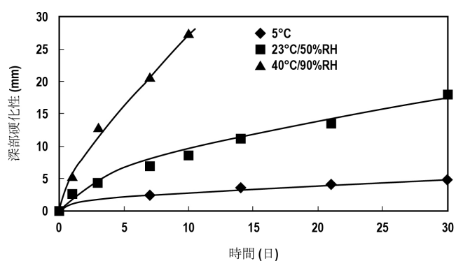
図 2: 深部硬化性
