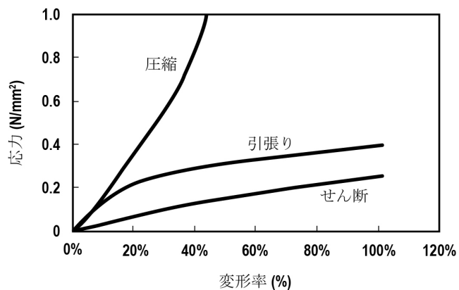
図 3: 変形率と応力の関係 (JIS A 1439 試験片)
