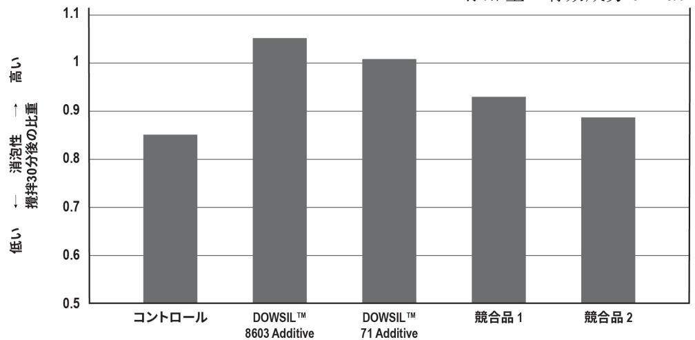
図 2: 同じく DOWSIL™ 8603 Additive を水性アクリルポリエステル塗料中に 0.2wt% を添加。ディゾルバーを使用して 5000 rpm で 3 分間高速攪拌混合した後に比重を測定。この評価結果は、DOWSIL™ 71 Additive や競合品と比較して DOWSIL™ 8603 Additive が優れた消泡性を提供することを示しています。
