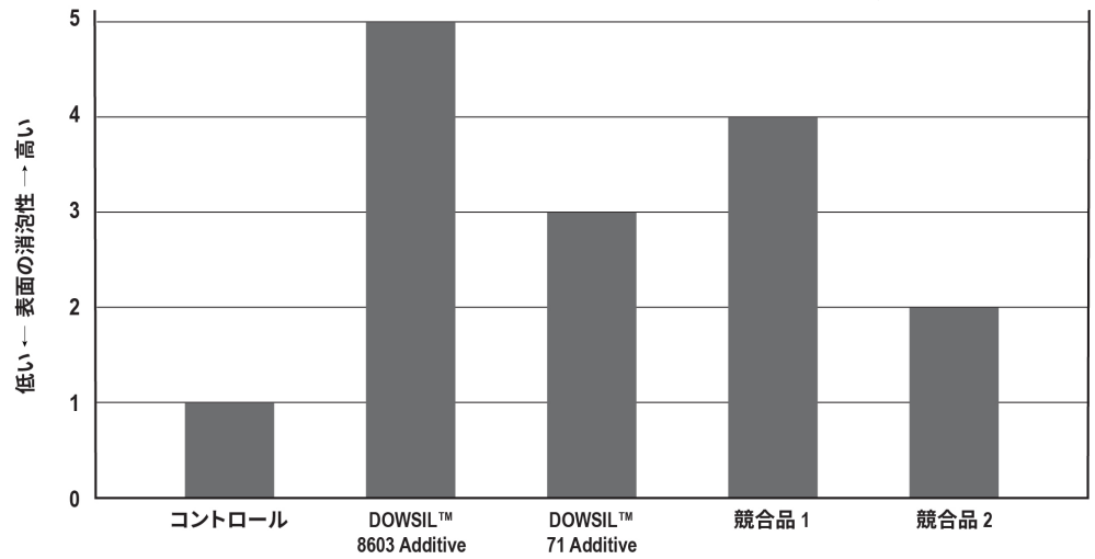
図 1: DOWSIL™ 8603 Additive を水性アクリルポリエステル塗料中に 0.2wt% を添加。同量の DOWSIL™ 71 Additive や競合品と比較して DOWSIL™ 8603 Additive は中毛ローラーで塗装時の塗膜表面の微細な泡を効果的に消します。
