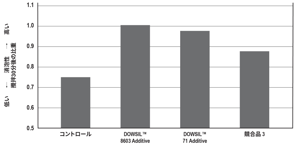
図 3: DOWSIL™ 8603 Additive の水性フレキシインキにおける消泡性。 DOWSIL™ 8603 Additive は 0.2wt% 添加でインキ用途でも優れた消泡剤として機能します。
