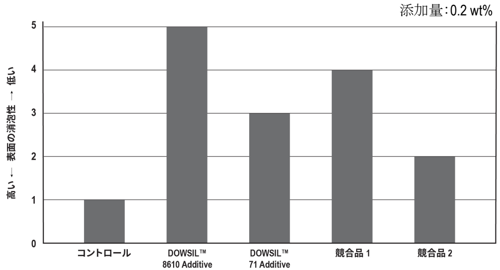
図 1: 0.2 wt%の DOWSIL™ 8610 Additive および DOWSIL™ 71 Additive を水系アクリルポリエステル塗料に添加。DOWSIL™ 8610 Additive は、中毛ローラーで塗布したときに発生する塗装表面の微細な泡を最も効果的に消します。
