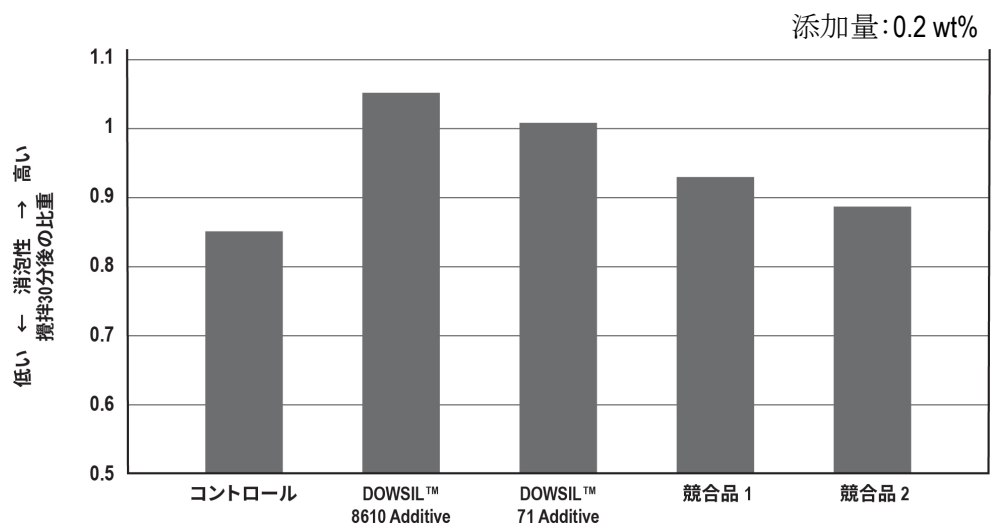
図 2: DOWSIL™ 8610 Additive および DOWSIL™ 71 Additive を水性アクリルポリエステル塗料に配合。ディゾルバーを使用して 5000 rpm で 3 分間高速攪拌混合した後のインク比重で消泡性を評価した。その結果、DOWSIL™ 8610 Additive が最も優れた消泡性を示しています。
