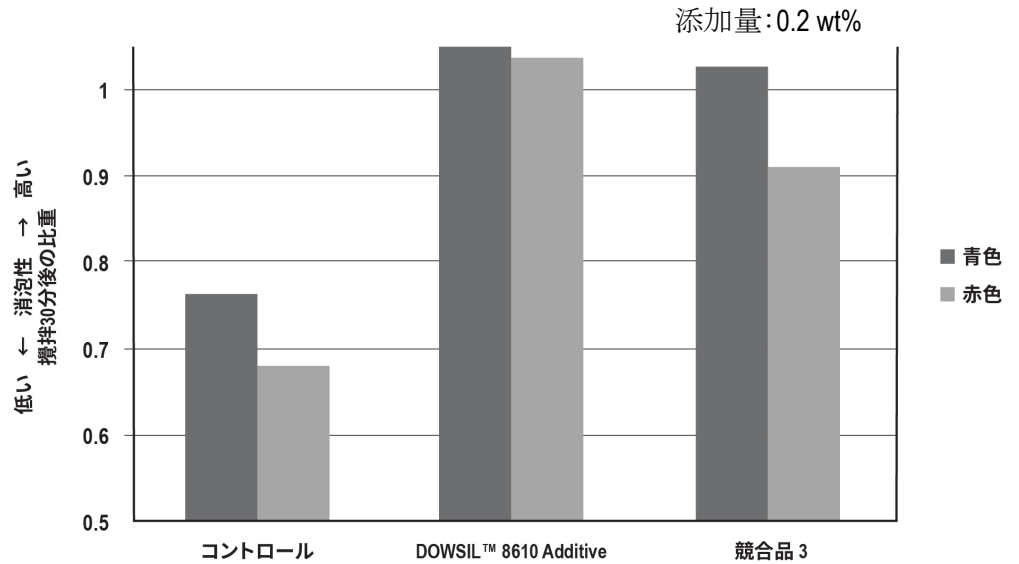
図 3: 2 種類の水性フレキシグラフィインキ (青と赤) における DOWSIL™ 8610 Additive の消泡性能。0.2 wt% 添加で DOWSIL™ 8610 Additive は、優れた消泡性能を発揮します。
