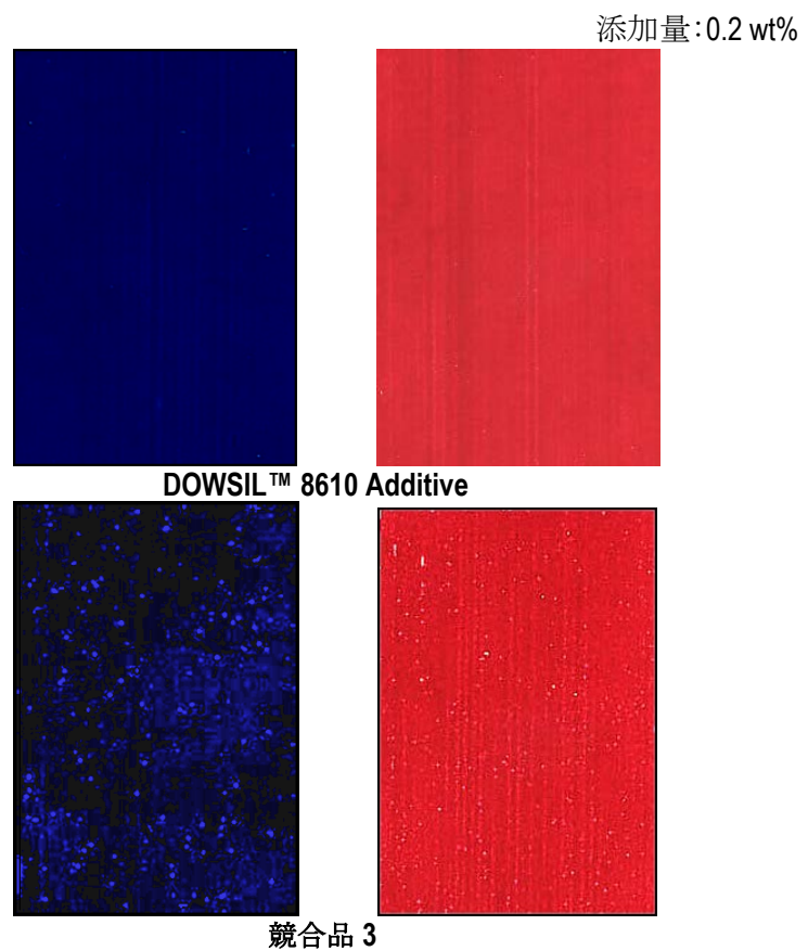
図 4: ポリエチレンラミネート塗工紙にウェット膜厚 18.3 ミクロンで塗工した水性フレキシインキの塗膜外観評価。この例は DOWSIL™ 8610 Additive が競合品 3 よりも塗膜欠陥のない優れた仕上がりを提供することを示しています。
