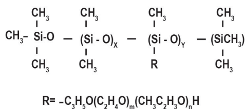
図 1 XIAMETER™ OFX-5220 の化学式
