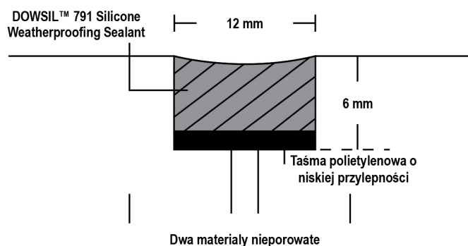
Rysunek 2: Złącze płytke.
