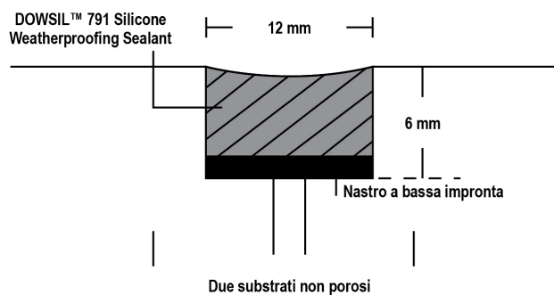
Figura 2: Junta Superficial
