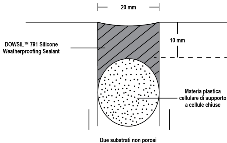
Figura 1: Junta Profunda
