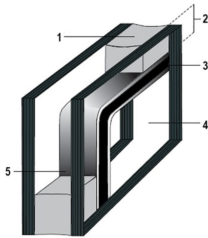
Figura 1: Corte característico de una unidad de acristalamiento aislante con doble barrera de estanqueidad.
