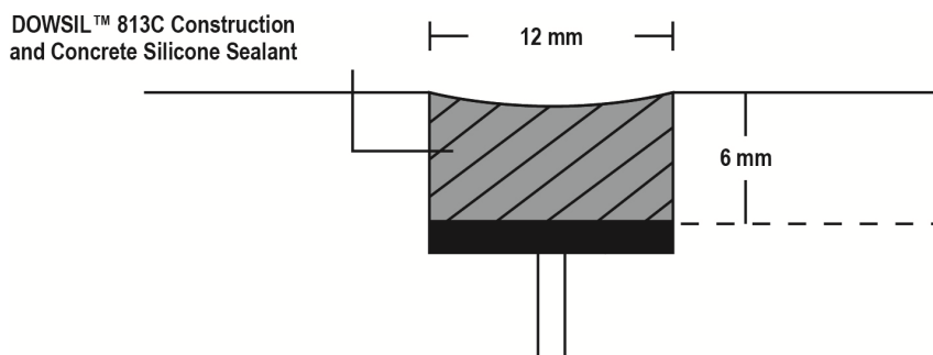
Figura 2: Junta Superficial
