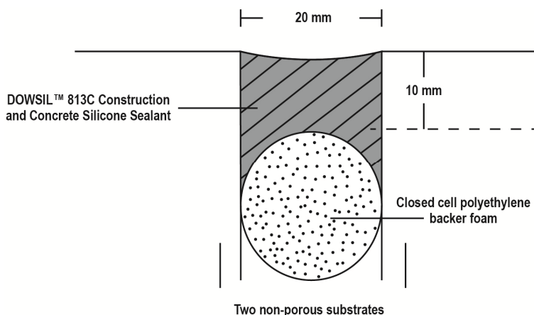
Figura 1: Junta Profunda
