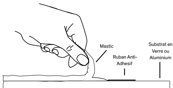
Test d'Adhérence par Pelage: Rupture Cohésive
