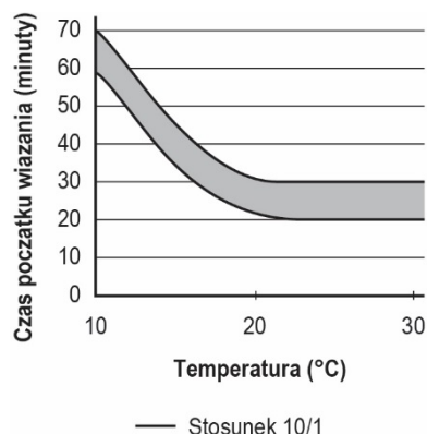
Rysunek 4: Szczeliwo DOWSIL™ 993 - zakres czasów początku wiązania.
