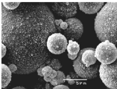
Figura 1: Imagen del DOWSIL™ 9701 Cosmetic Powder en un microscopio electrónico de barrido.
